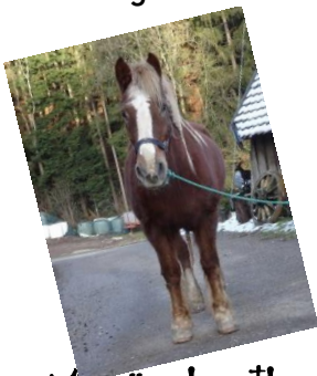
Leda 1991-2019
